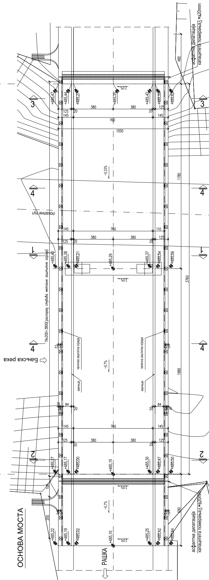
Прилог 2 – Основа моста - новопроектвано стање
