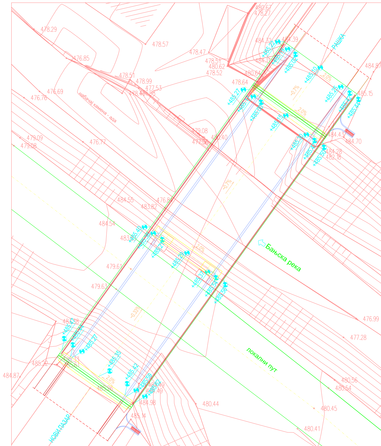
Прилог 1 – Ситуациони план - новопројектовано стање
