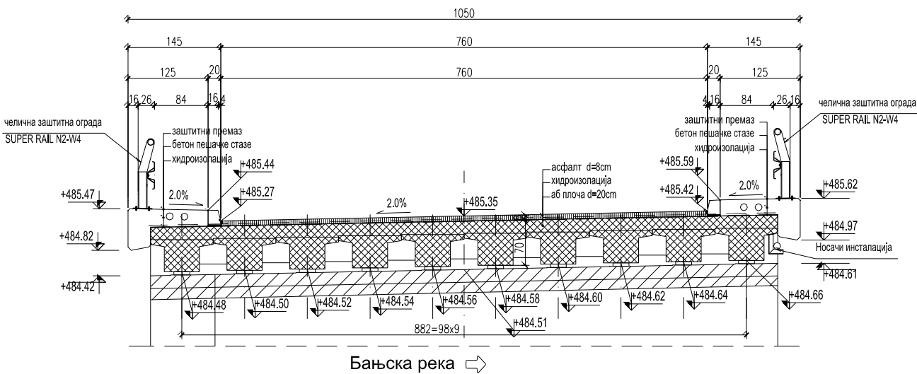
Прилог 3 – Попречни пресеци - новопроектовано стање
